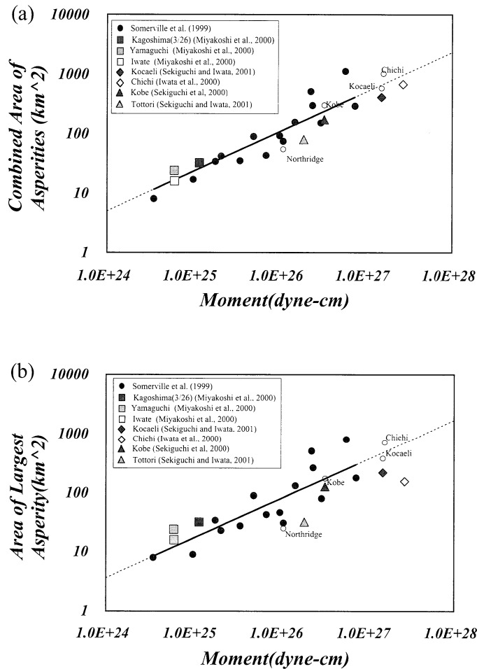
図 17 震源インバージョンの結果を基に抽出された特性化震源モデルのアスぺリティ総面積 (a) および最大アスぺリティ面積と地震モーメントの関係 (b) (Miyakoshi, 2001 私信による). 黒線は Somerville et al. (1999) によって傾きを 2/3 に固定して得られた回帰式を示す. 広い周波数帯域における強震動シミュレーションから推定された最適震源モデルが白丸印で示される.
