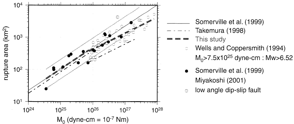
図 7 断層面積と地震モーメントの関係。
