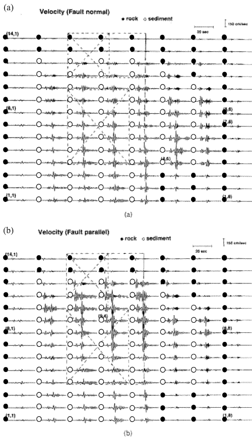
図 19 正断層震源解(菊地ほか, 1999)を基に構築された特性化震源モデルを用いて計算された1948年福井地震の強震動。(a)は断層直交成分,(b)は断層平行成分を示す。計算領域は長方形の実線で囲まれた領域(1,1)~(14,8)のグリッドに分けられており,●は岩盤点,○は堆積層上の点に対応する。破線でXマークが付されたところは2つのアスペリティの地表投影に対応する。(入倉・釜江, 1999による)
