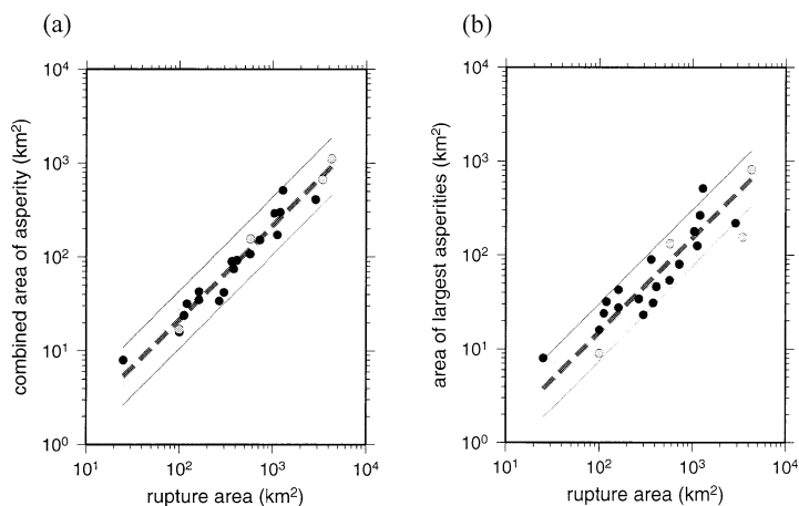
図 9 (a) アスペリティの総面積と断層面積の関係。
