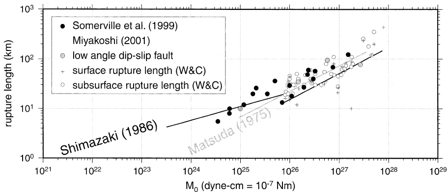
図 3 断層長ささと地震モーメントの関係。
